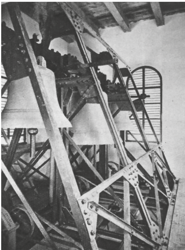
Kostelní zvony s elektrickým pohonem
